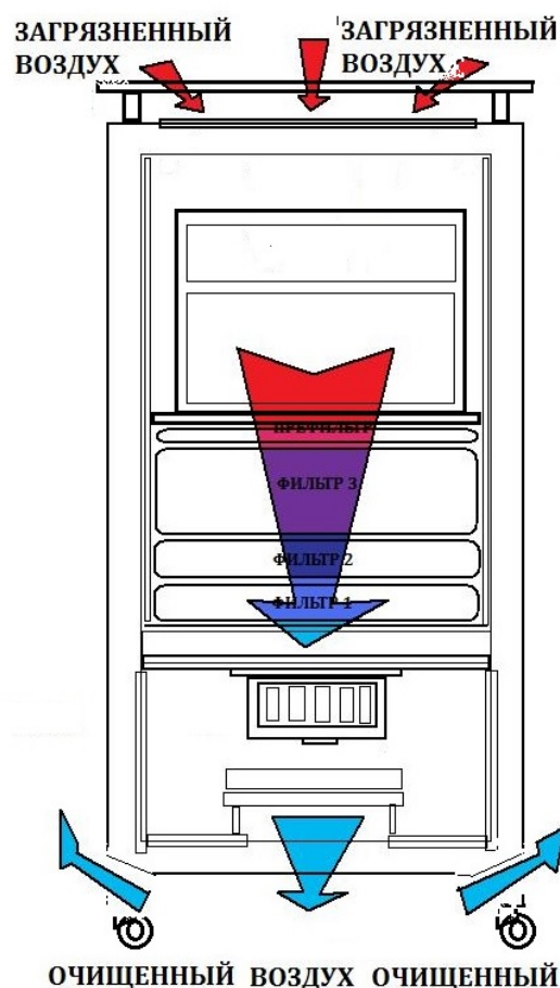
схема принципа работы воздухоочистителя
