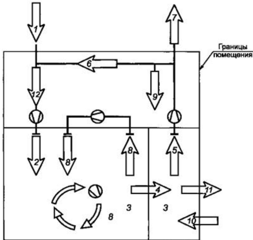
Рисунок 1 - Типы потоков воздуха. Номера позиций соответствуют таблице 2
