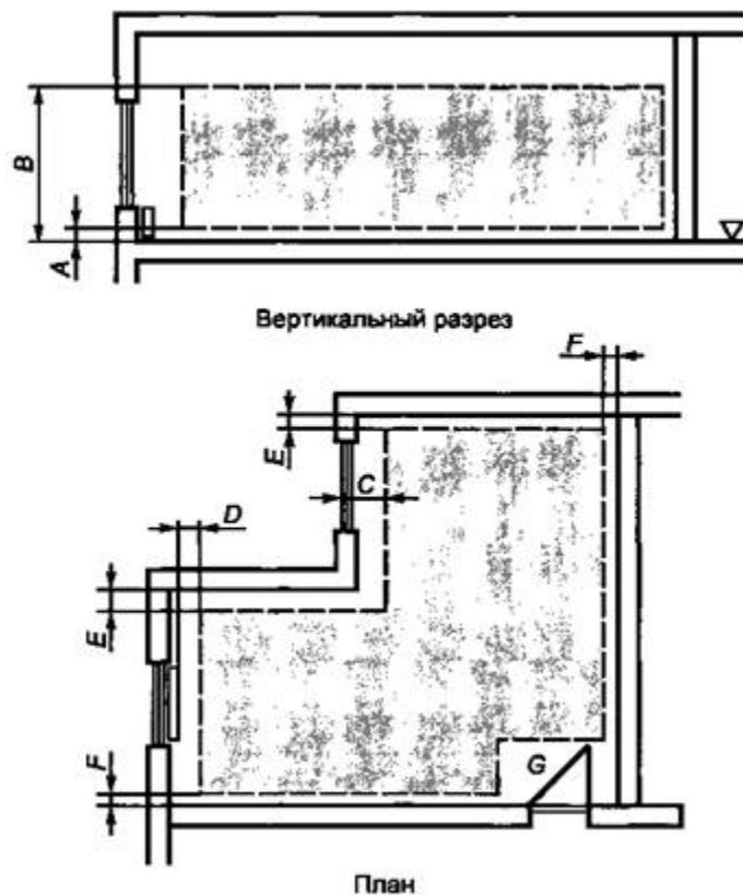
Рисунок 2 - Пример рабочей зоны (выделена фоном)
